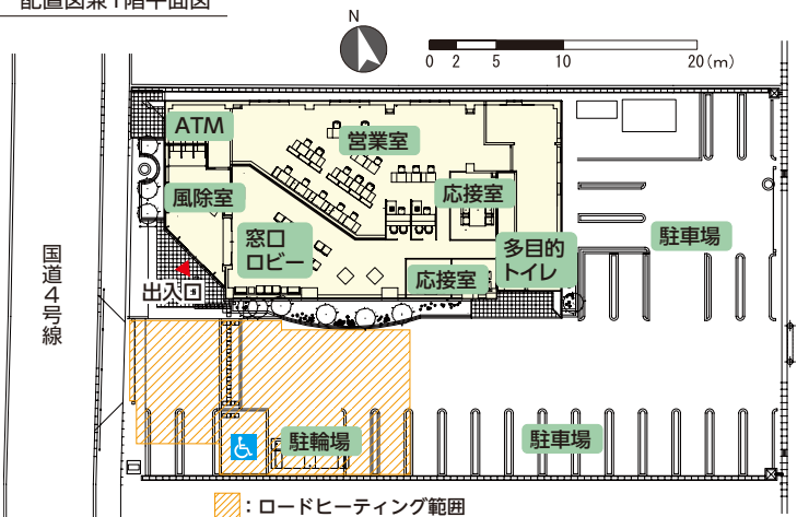
配置図兼1階平面図
